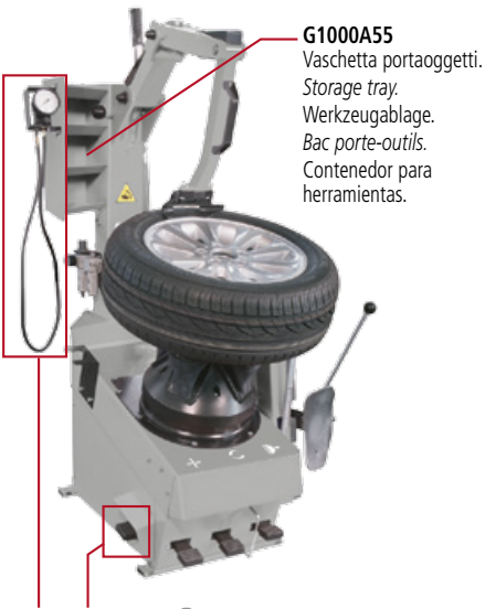
G1000A51 G800A120 Variante gonfiaggio con comando a pedale, manometro e valvola bilanciatrice. Assemblaggio in fabbrica. Pedal activated inflator, gauge and balancing valve. Factory installed. Pedalgesteuerter Reifenfüller mit Manometer und Druckregler. Werksseitig montiert. Variante gonflage commande à pédale, manomètre et valve de dosage. Monté en usine. Suplemento para inflado con mando a pedal, manómetro y válvula repartidora. Montado en fabrica.
